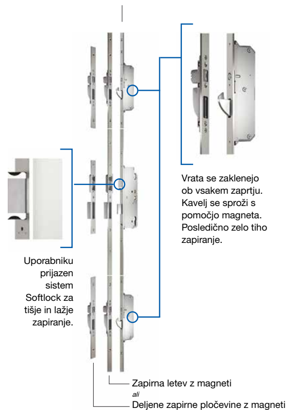
Ključavnica (Inox) 3500 s kavlji in magnetnim sprožilcem
