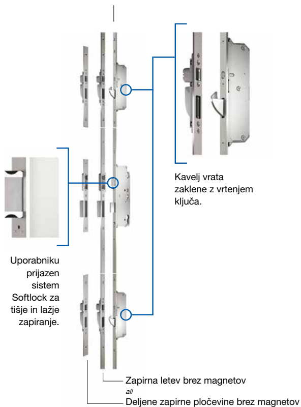
Ključavnica 2500 s kavlji na ročno zaklepanje
