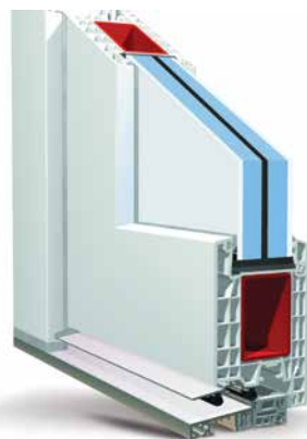
PVC profil 76 s klasičnim pragom
