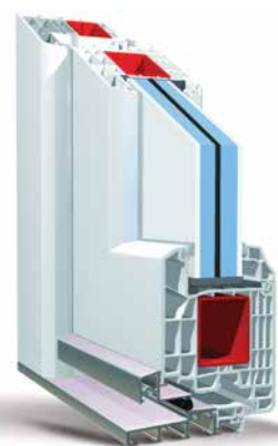
PVC profil 88 s klasičnim pragom
